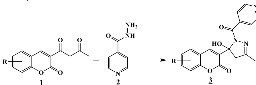
Schéma 1: Synthèse des molécules hybrides d'isonicotinoyl-pyrazolylcoumarine 3
